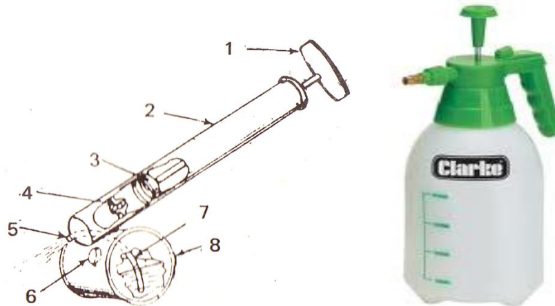
Gambar 48. Alat semprot jenis Atamozer
