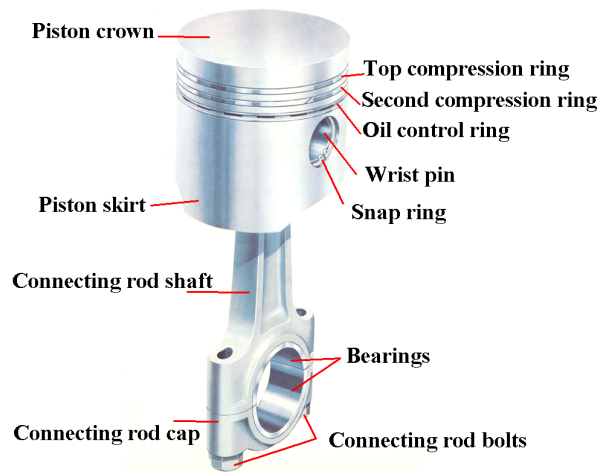
Gambar 102. Torak dan kelengkapannya
