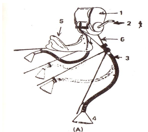
Gambar 52. Alat Penghembus Ditarik Hewan
