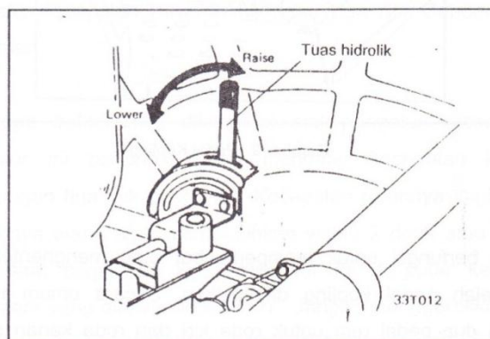
Gambar 128. Tuas hidrolik
