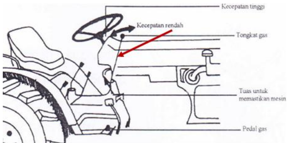
Gambar 136. Tuas gas
