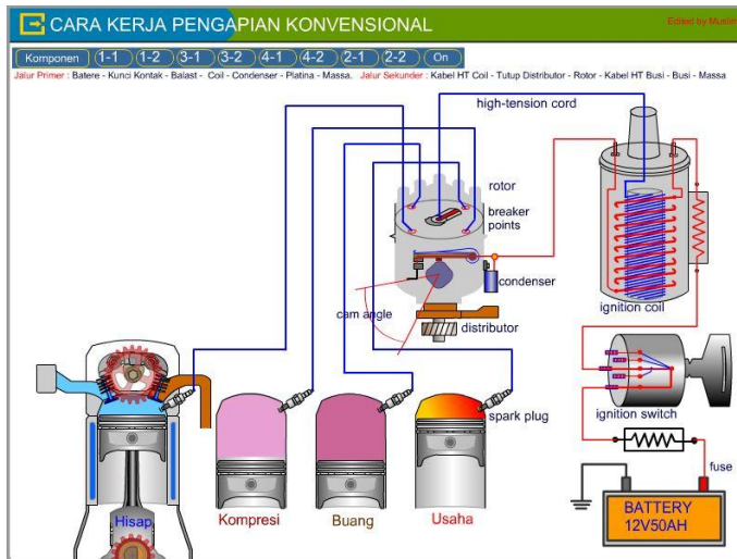
Gambar 114. Sistem Pengapian (Motor Bensin)
