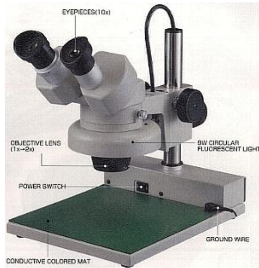
Gambar 77. Mikroskop Stereo
