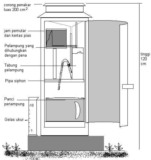
Gambar 157. Bagian-bagian Alat Penakar Hujan (Hellman)
