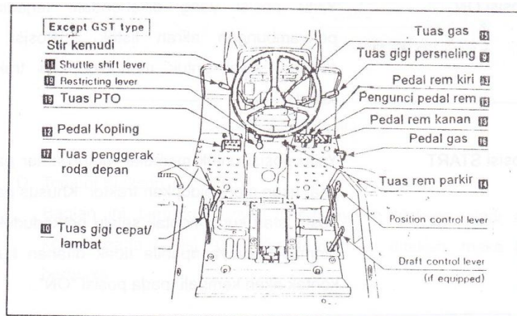
Gambar 121. Alat-alat kontrol
