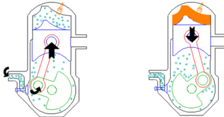
Langkah isap dan kompresi
