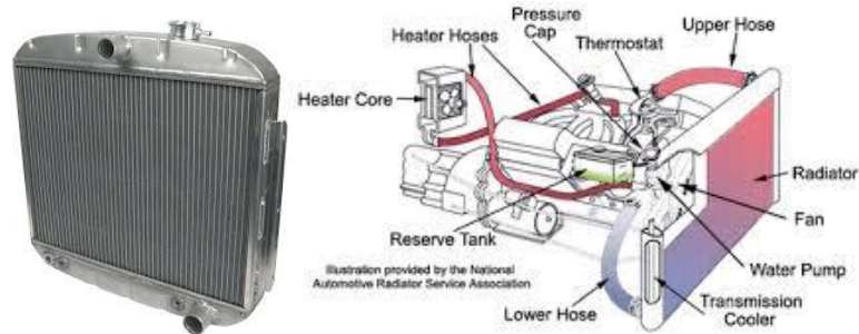
Gambar 113. Motor dengan sistem pendingin radiator
