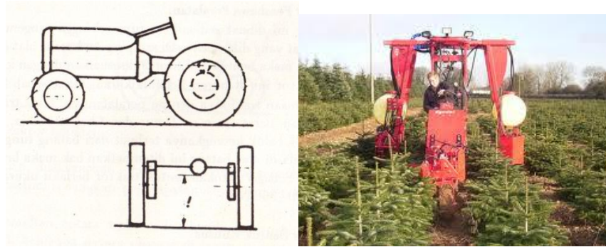
Gambar 15. Traktor Portal
