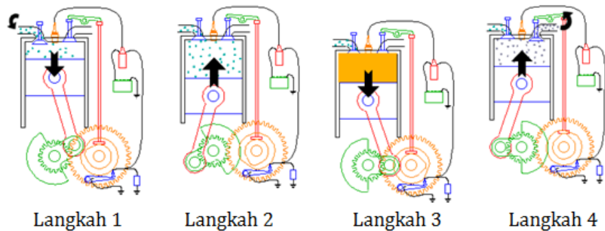
Gambar 162. Langkah-langkah Pada Motor 4 Tak
