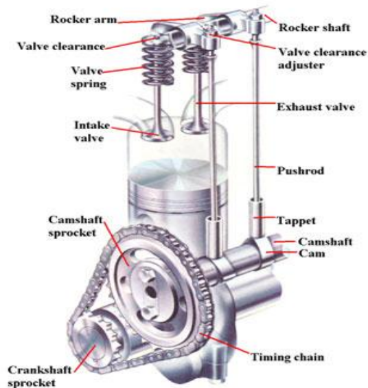
Gambar 107. Mekanisme Katup
