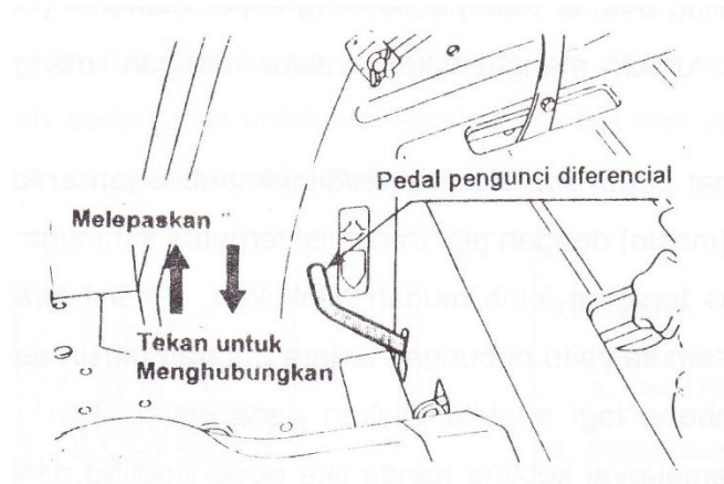
Gambar 127. Pedal pengunci garden
