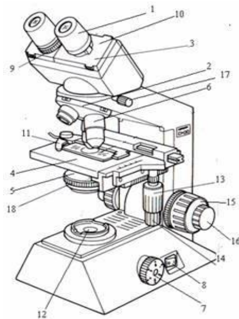
Gambar 152. Bagian-bagian Mikroskop
