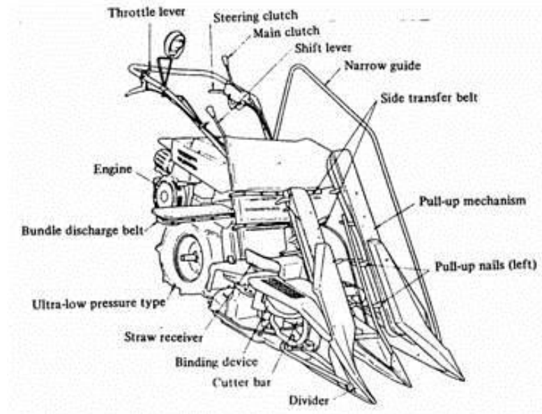
Gambar 150. Bagian-bagian alat panen padi (Binder)
