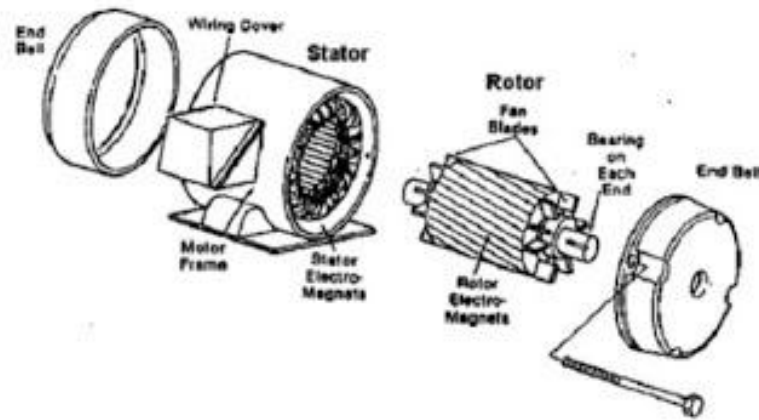
Gambar 6. MotorInduksi.
