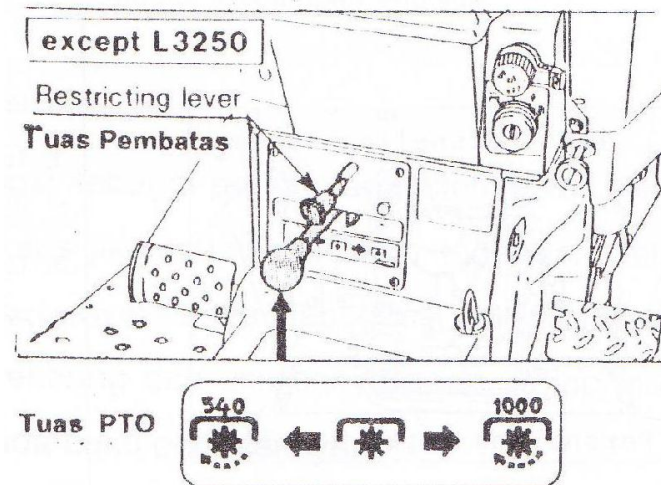
Gambar 126. Tuas PTO
