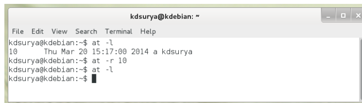
Gambar 43. Contoh penerapan parameter pada perintah at
