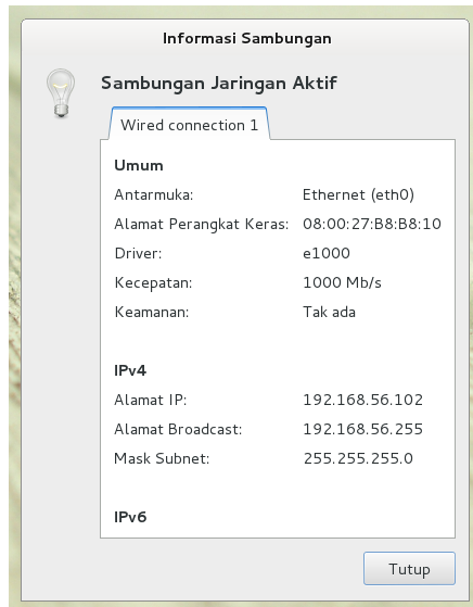
Gambar 25. Informasi koneksi dari jaringan terpilih
