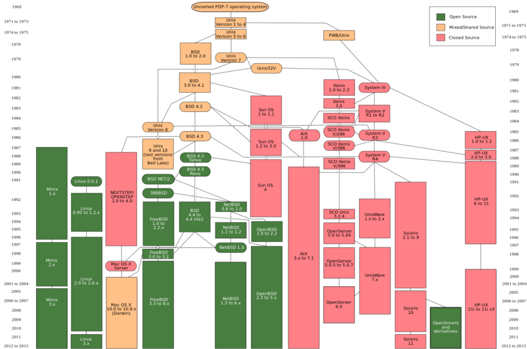
Gambar 5. Sejarah perkembangan sistem operasi UNIX dan turunannya
