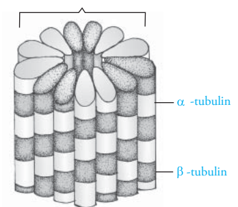
Gambar 1.22 Susunan alpha dan beta tubulin pada mikrotubulus
