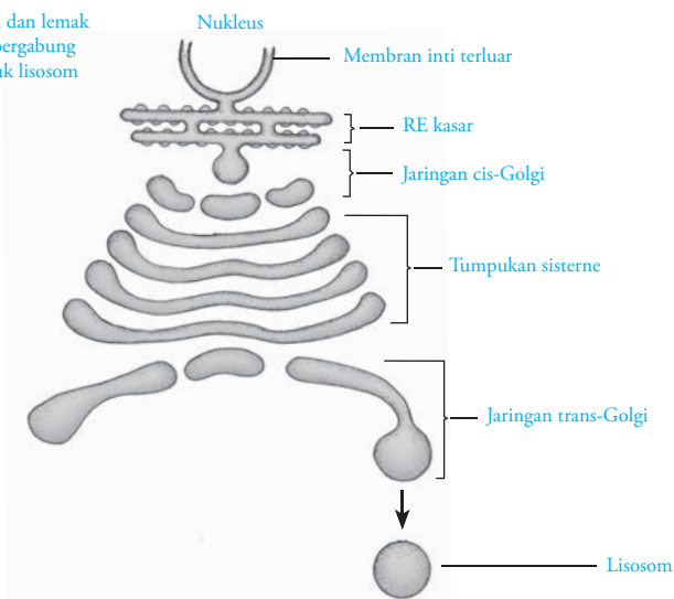
Gambar 1.11 Aparatus Golgi dan hubungannya dengan nukleus, retikulum endoplasma dan liso-
