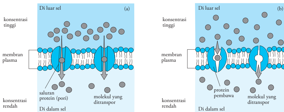
Gambar 1.28 Difusi zat (a) dipermudah dengan protein (b) terfasilitasi dengan protein pembawa
