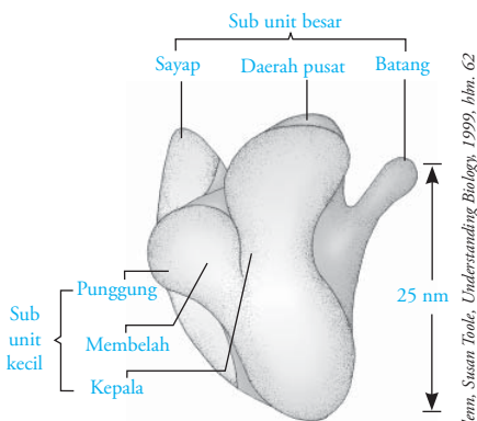
Gambar 1.19 Struktur ribosom
