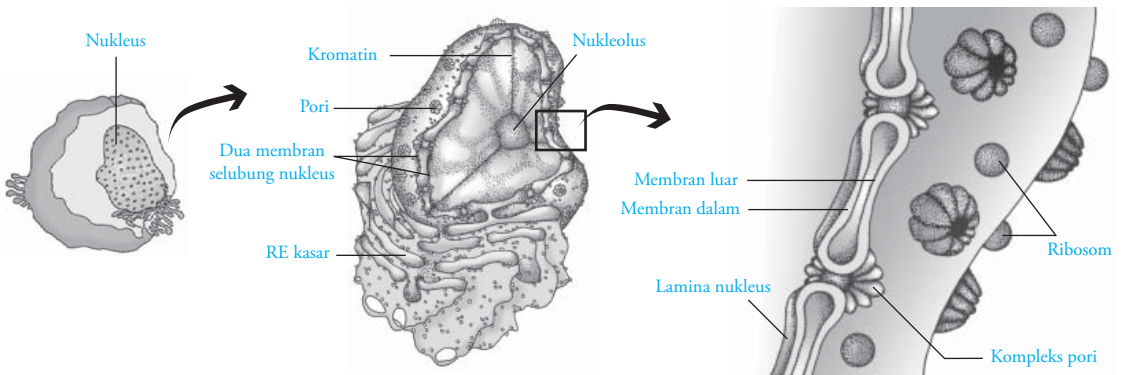
Gambar 1.7 Struktur nukleus
