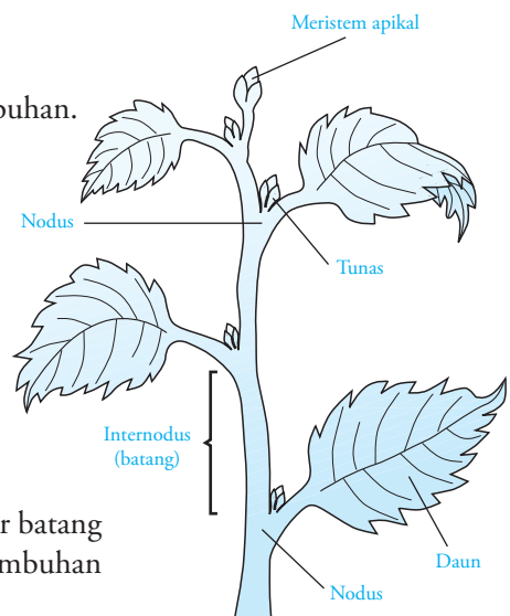
Gambar 2.24 Bagian-bagian batang
