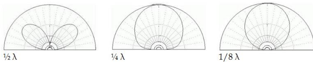
Gambar 6.9. Pola radiasi antenna dipole \frac{1}{2} \lambda untuk beberapa ketinggian antena
