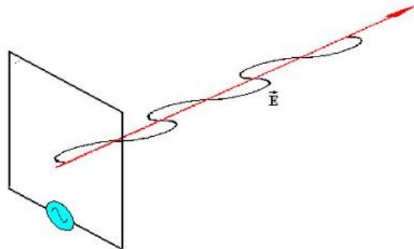
Gambar 2.6. Polarisasi Horizontal
