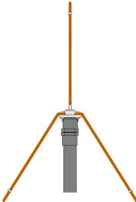
Gambar 7.21. Bentuk akhir antena ground plane vertikal
