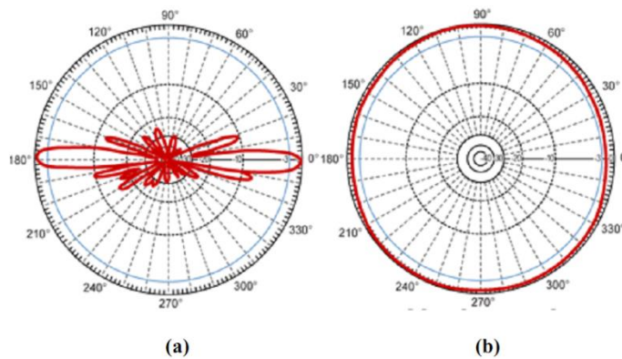
Gambar 6.6. Bentuk pola radiasi gelombang antena Omnidirectional
