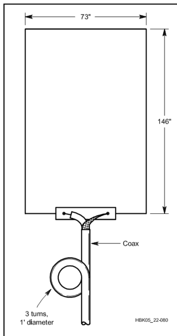
Gambar 10.7. Rancangan antena Loop persegi panjang
