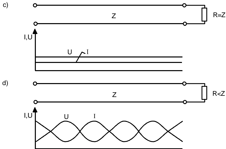
Gambar 5.7. Kondisi gelombang dengan beban diujung penghantar
