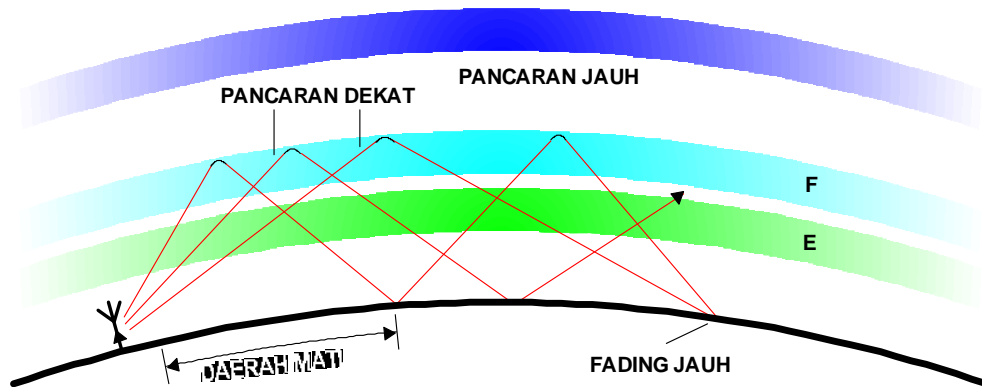
Gambar 1.6. Daerah Mati
