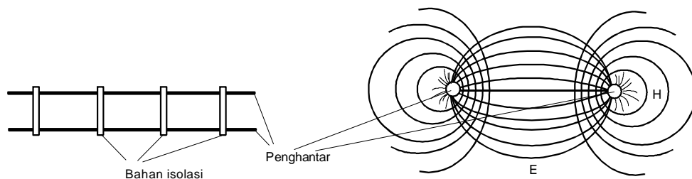
Gambar 5.8. Gambaran gelombang di kabel simetris
