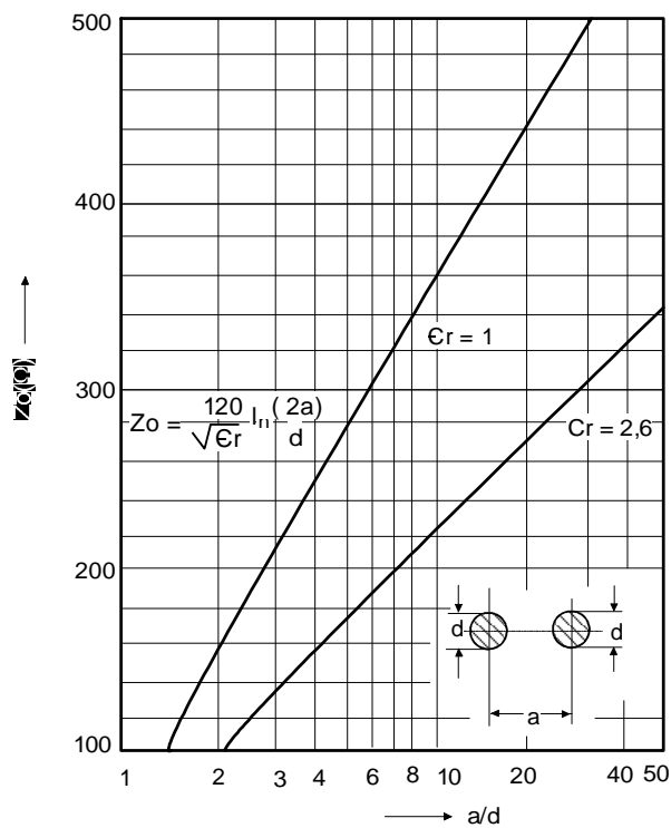
Gambar 5.9. Grafik Impedansi
