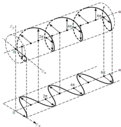
Gambar 2.1. Polarisasi Linier
