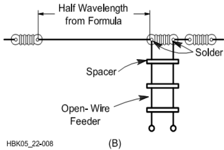
Gambar 7.7. Pengumpan pada Antena Dipole multiband
