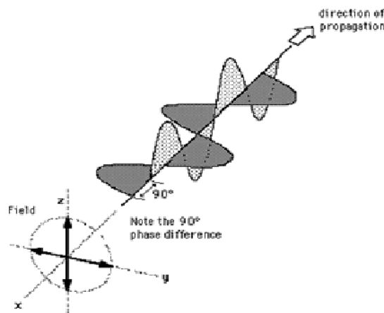
Gambar 2.7. Polarisasi Circular
