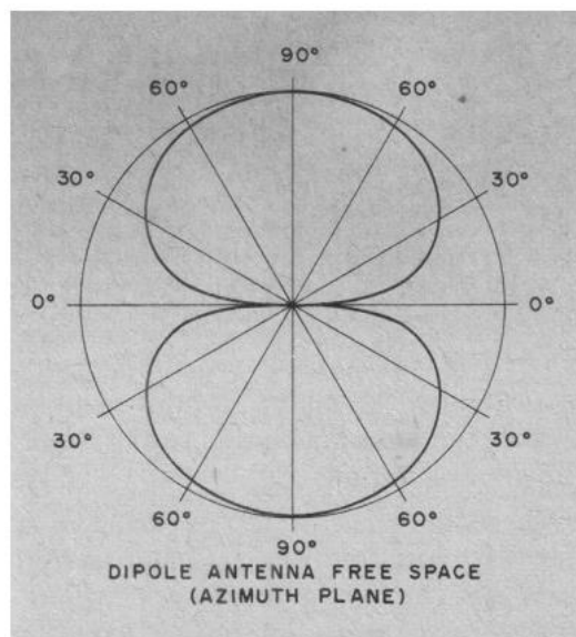
Gambar 8.3. Arah pancaran antena Dipole
