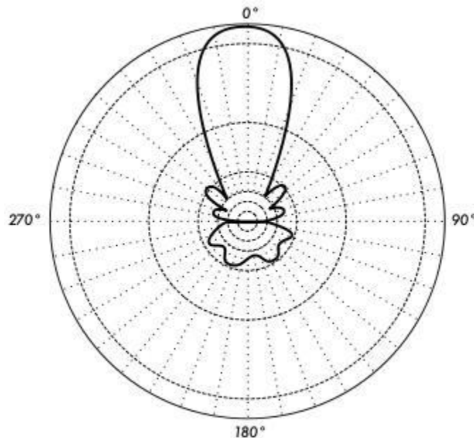
Gambar 6.1. Dimensi pola radiasi
