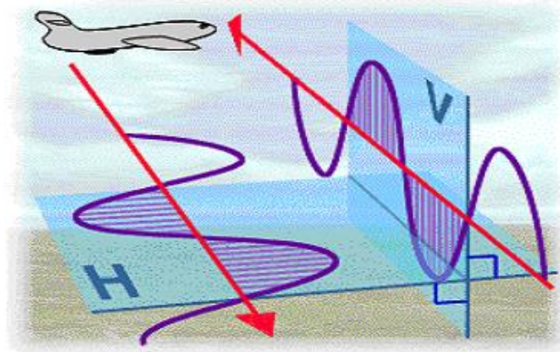
Gambar 2.8. Polarisasi Cross
