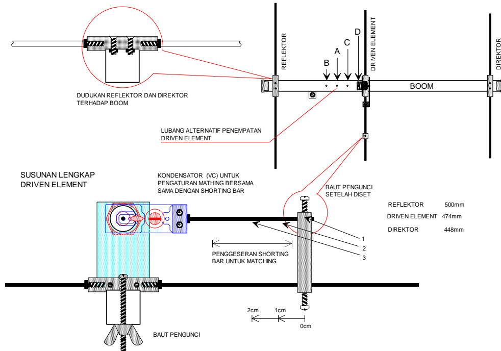
Gambar 9.12. Susunan pemasangan elemen antenna
