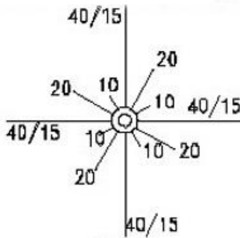
Gambar 3.4. Peletakan Radial Ground
