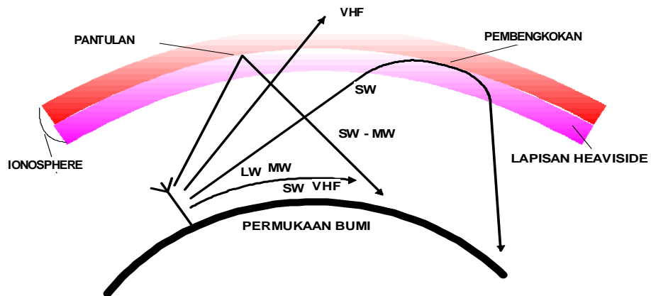
Gambar 1.2. Pemantulan Gelombang
