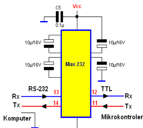
Gambar 4.15 Konversi tegangan RS232-TTL
