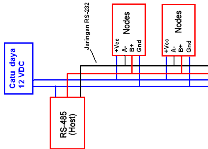
Gambar 4.2. Komunikasi EIA-485 untuk Pengirim Cerdas.
