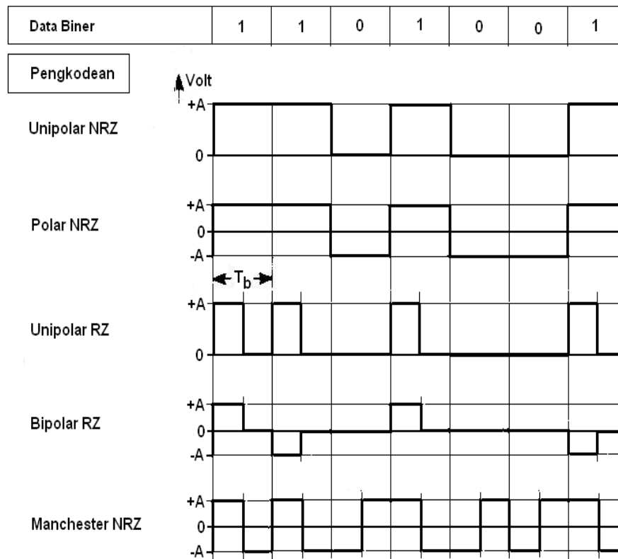
Gambar 1.11 Pengkodean bit biner ( line-code ).
