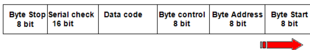
Gambar 1.19. Frame pesan HDLC
