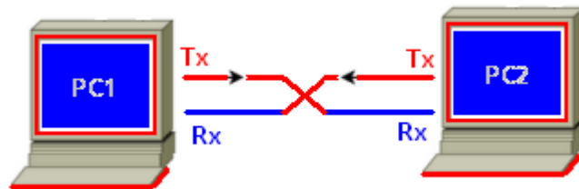
Gambar 4.12. Koneksi 2 komputer melalui Tx/Rx pada RS232.
