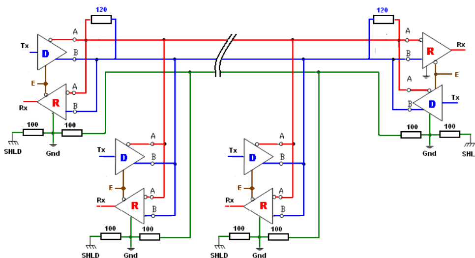
Gambar 4.19. Jaringan RS-485
