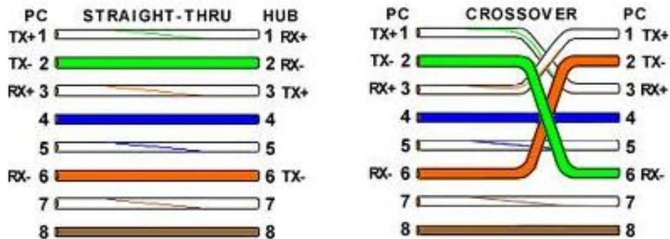
Gambar 2.8. Dua Jenis Konfigurasi Kabel UTP Straight-Thru dan Cross-Over
