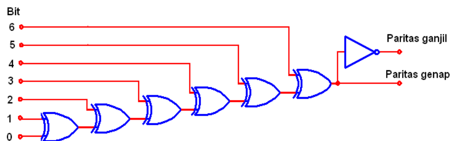
Gambar 1.14. Rangkaian pembangkit paritas
