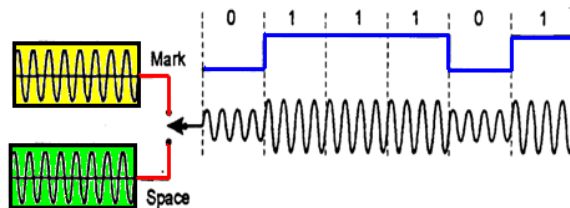
Gambar 4.28. Modulasi ASK
