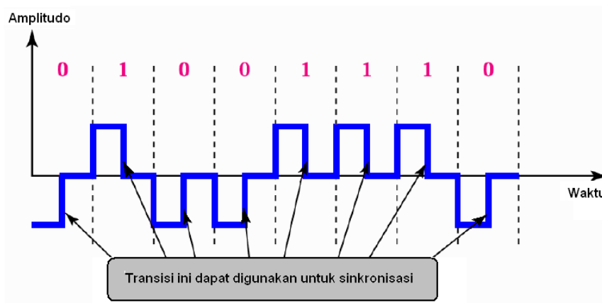
Gambar 1.8. Diagram pulsa pengkodean RZ
